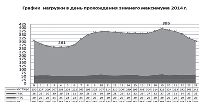
График совмещенной нагрузки «Центрального энергорайона» на день прохождения зимнего максимума в 2014 году
