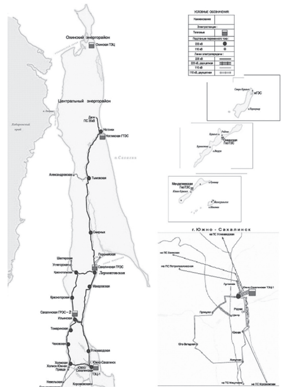
Схема развития электроэнергетики Сахалинской области на 2015 – 2019 годы
